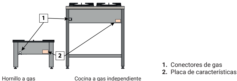
Figura 15. Vista trasera del dispositivo.
