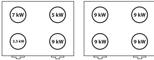
Figura 6. Colocación de los quemadores en cocinas con cuatro quemadores (esquemático)
