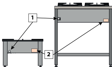
Rysunek 15. Widok od tyłu na urządzenie.
