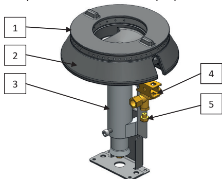
Figure 16. Construction du brûleur basée sur l'exemple du brûleur de 7 kW.
