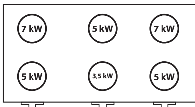
Obrázok 7. Umiestnenie horných horákov na sporáku so šiestimi horákmi (schematicky)
