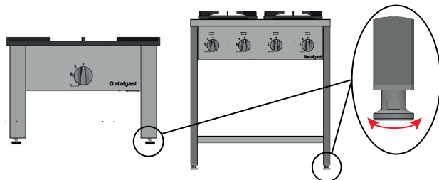
Obrázek 14. Vyrovnávání zařízení
