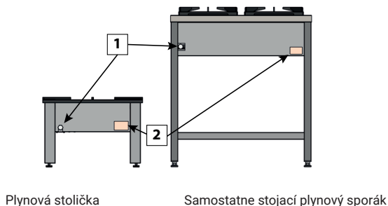
Obrázok 15. Pohľad zo zadnej strany zariadenia.
