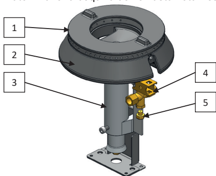
Figura 16. Diseño del quemador sobre el ejemplo de un quemador de 7 kW.
