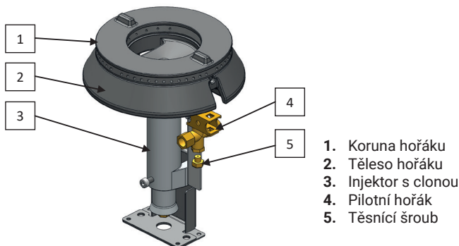
Obrázek 16. Konstrukce hořáku na příkladu 7kW hořáku.
