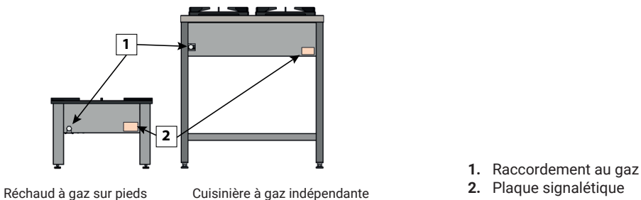
Figure 15. Vue sur l'arrière de l'appareil.
