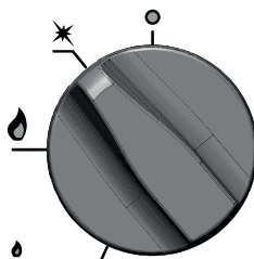
Figura 9. Ajuste del mando en el que solo el quemador piloto cuenta con flujo de gas
