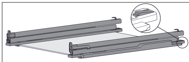
Fig. 41 Płyta szklana z szynami i elementami mocującymi
